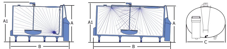
Vanaf model O 2000, tank uitgerust met sproeibolreiniging (met demontabele leiding).
